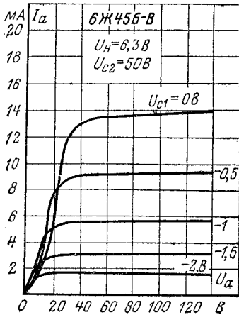
Анодные характеристики.
