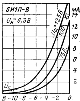
Анодно-сеточные характеристики.
