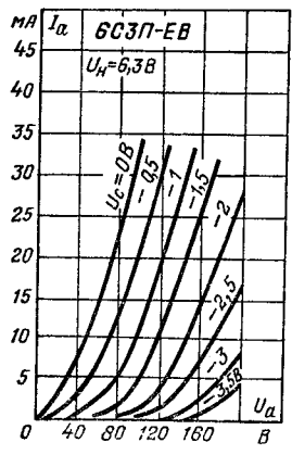
Анодные характеристики.
