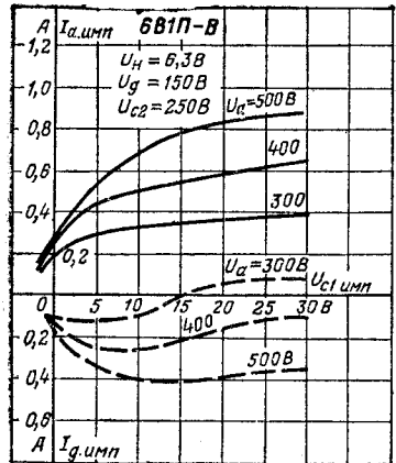
Импульсные анодно-сеточные (сплошные) и анодно-катодные (пунктирные) характеристики.
