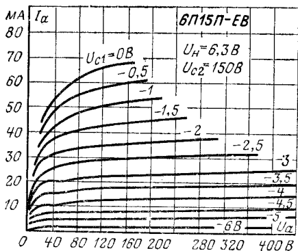
Анодные характеристики.
