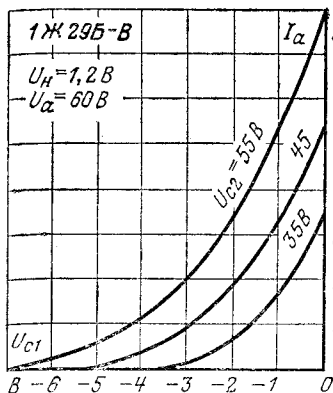
Анодно-сеточные характеристики.
