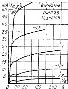
Анодные характеристики.
