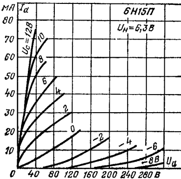
Анодные характеристики.
