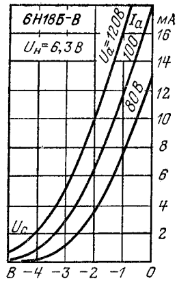
Анодно-сеточные характеристики.
