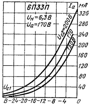
Анодно-сеточные характеристики.
