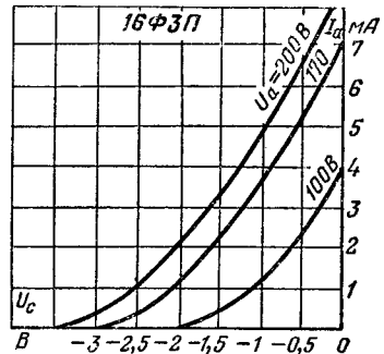
Анодно-сеточные характеристики триодной части.
