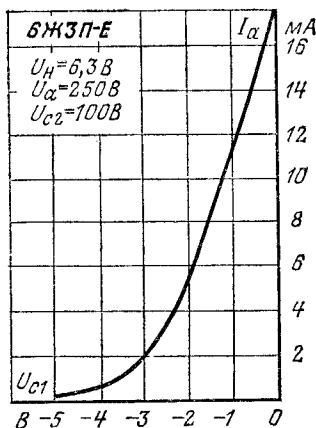
Анодно-сеточная характеристика.
