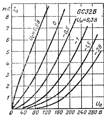
Анодные характеристики.
