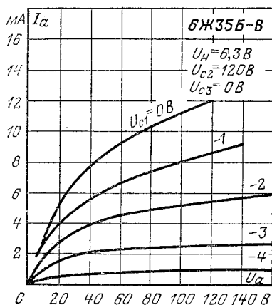
Анодные характеристики.
