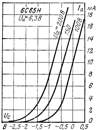
Анодно-сеточные характеристики.
