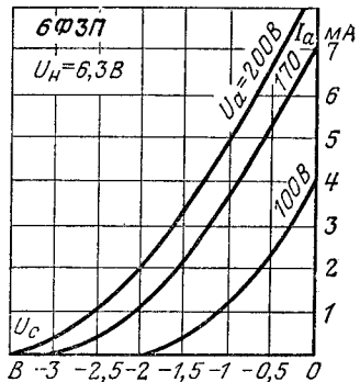
Анодно-сеточные характеристики триодной части.
