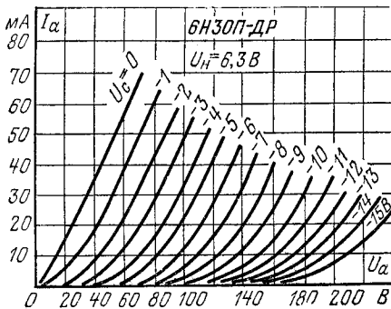
Анодные характеристики.
