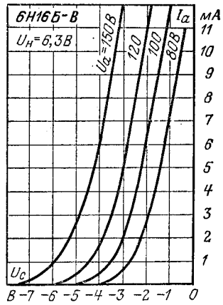
Анодно-сеточные характеристики.
