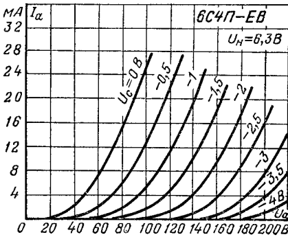
Анодные характеристики.
