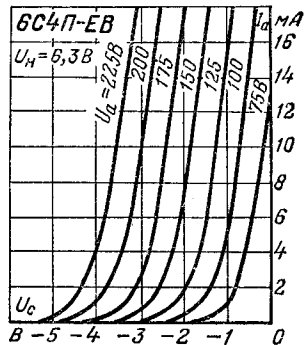
Анодно-сеточные характеристики.
