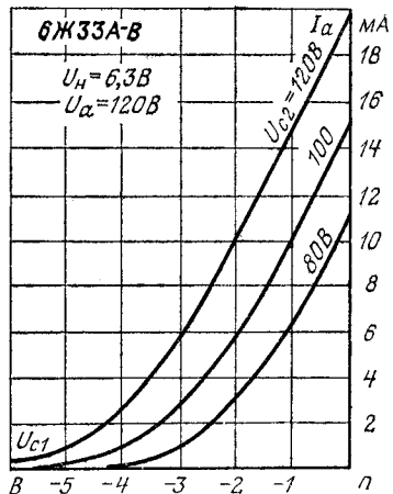
Анодно-сеточные характеристики.
