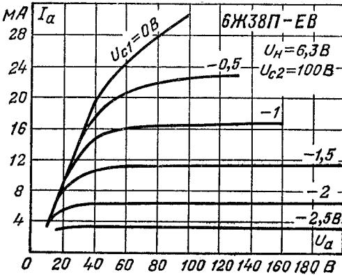
Анодные характеристики.
