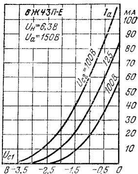
Анодно-сеточные характеристики.
