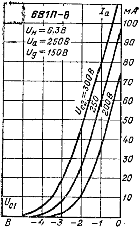
Анодно-сеточные характеристики.
