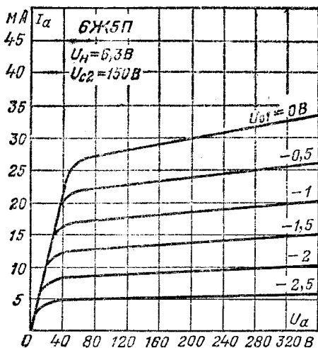
Анодные характеристики.
