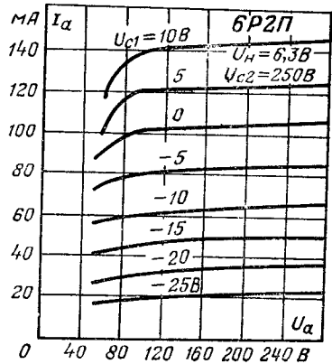
Анодные характеристики.
