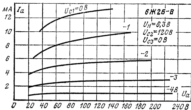
Анодные характеристики.
