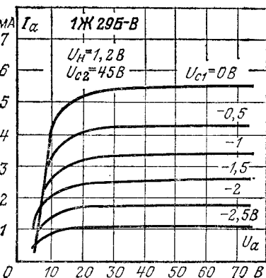
Анодные характеристики.
