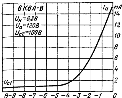
Анодно-сеточная характеристика.
