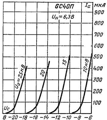
Анодно-сеточные характеристики.
