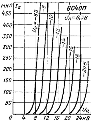
Анодные характеристики.
