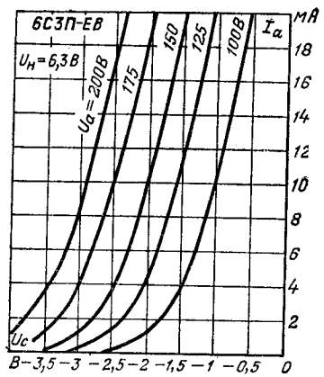
Анодно-сеточные характеристики.
