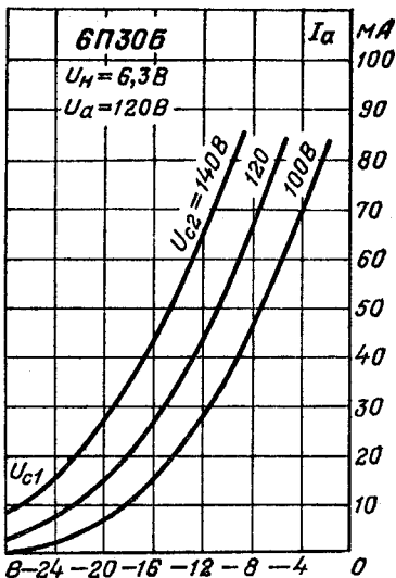
Анодно-сеточные характеристики.
