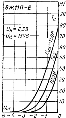
Анодно-сеточные характеристики.
