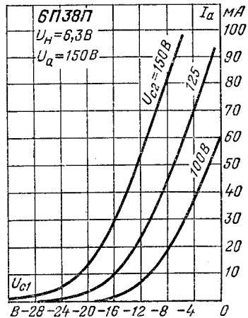
Анодно-сеточные характеристики.
