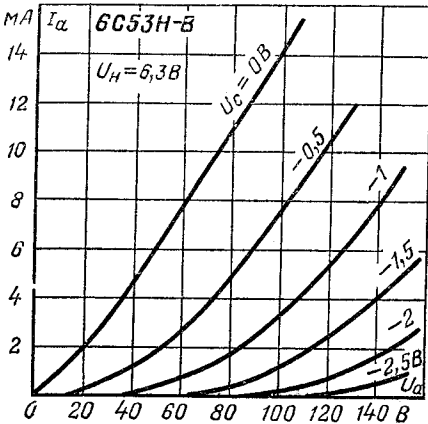
Анодные характеристики.
