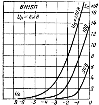
Анодно-сеточные характеристики.
