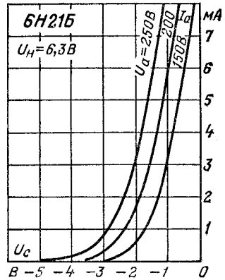
Анодно-сеточные характеристики.
