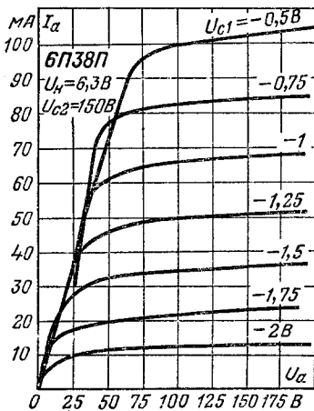
Анодные характеристики.
