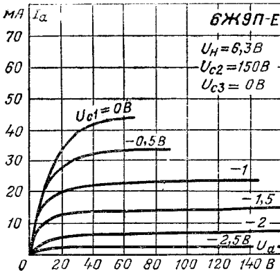
Анодные характеристики.
