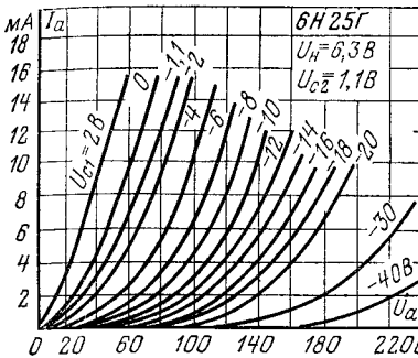
Анодные характеристики.
