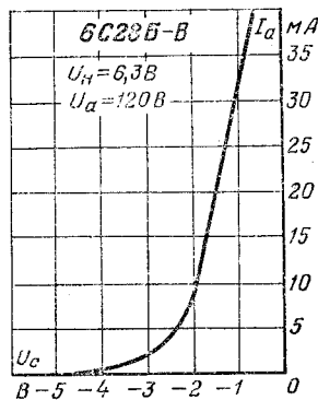
Анодно-сеточные характеристики.
