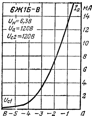
Анодно-сеточная характеристика.
