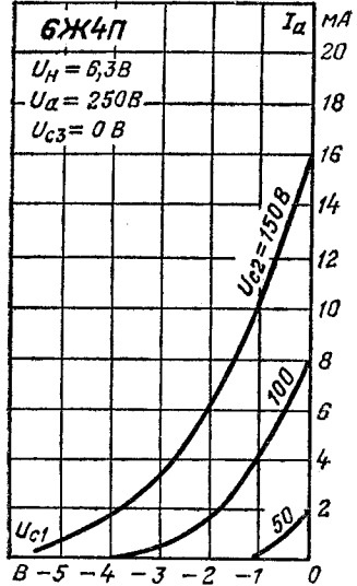
Анодно-сеточные характеристики.
