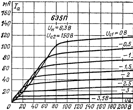
Анодные характеристики.
