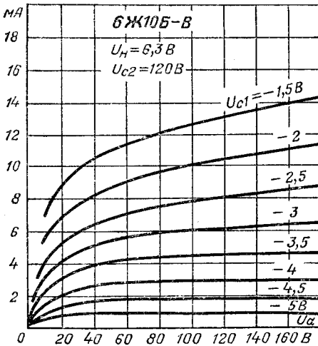
Анодные характеристики.
