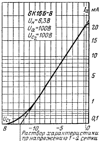
Анодно-сеточная характеристика.
