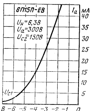
Анодно-сеточная характеристика.
