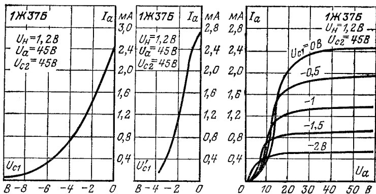
Анодно-сеточная характеристика по 1-й сетке (сетки C'_1 и C''_1 соединены).
