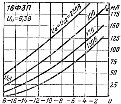
Анодно-сеточные характеристики пентодной части.
