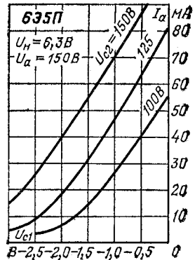
Анодно-сеточные характеристики.
