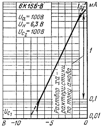
Анодно-сеточная характеристика.
