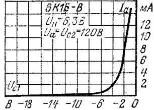
Анодно-сеточные характеристики.
