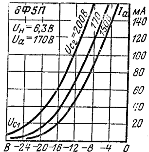
Анодно-сеточные характеристики пентодной части.
