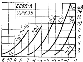
Анодно-сеточные характеристики.
