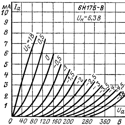
Анодные характеристики.
