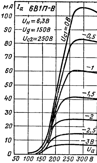
Анодные характеристики.
