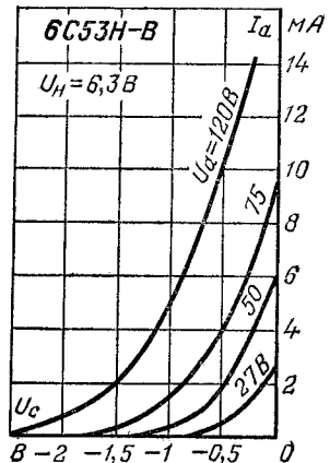
Анодно-сеточные характеристики.
