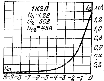
Анодно-сеточные характеристики.
