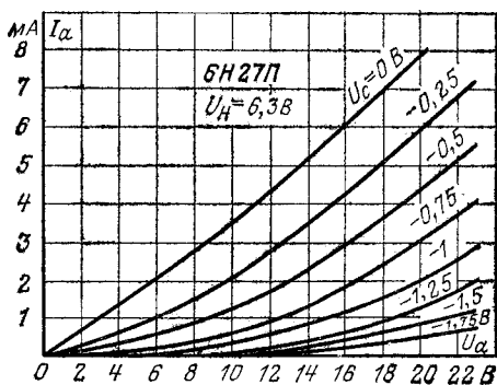
Анодные характеристики.
