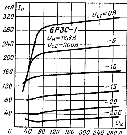
Анодные характеристики.
