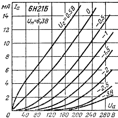
Анодные характеристики.
