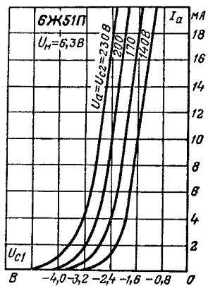
Анодно-сеточные характеристики.
