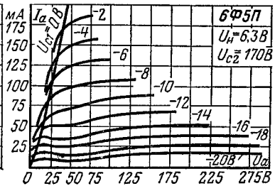
Анодные характеристики пентодной части.
