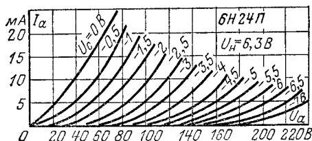
Анодные характеристики.
