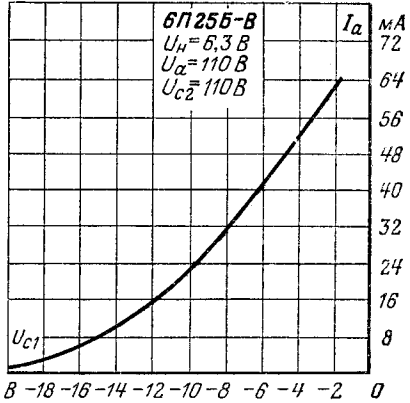
Анодно-сеточная характеристика.
