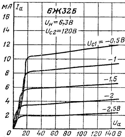
Анодные характеристики.
