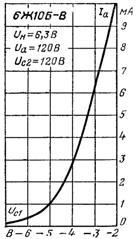
Анодно-сеточная характеристика.
