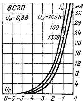
Анодно-сеточные характеристики.
