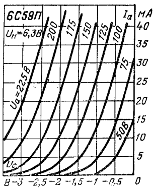
Анодно-сеточные характеристики.
