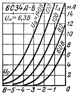
Анодно-сеточные характеристики.
