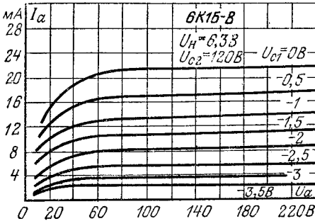
Анодные характеристики.
