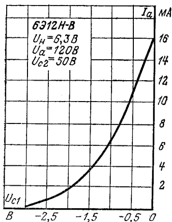
Анодно-сеточные характеристики.
