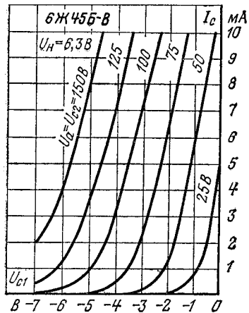
Анодно-сеточные характеристики.
