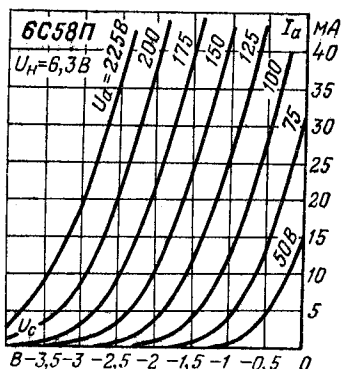
Анодно-сеточные характеристики.
