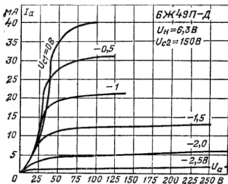
Анодные характеристики.
