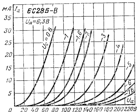
Анодные характеристики.
