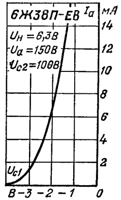
Анодно-сеточная характеристика.
