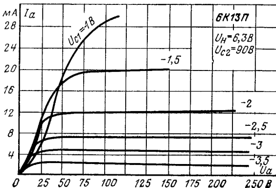
Анодные характеристики.
