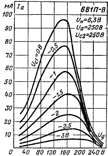
Анодно-катодные характеристики.
