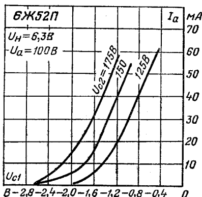
Анодно-сеточные характеристики.
