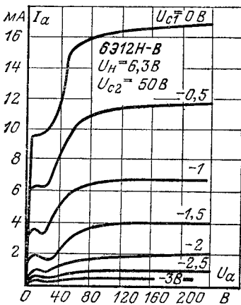
Анодные характеристики.
