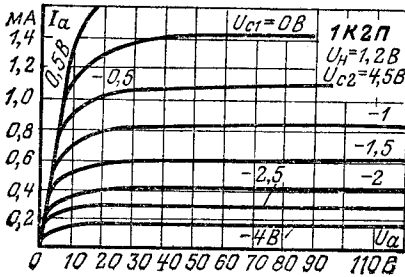
Анодные характеристики.
