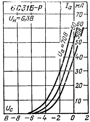
Анодно-сеточные характеристики.
