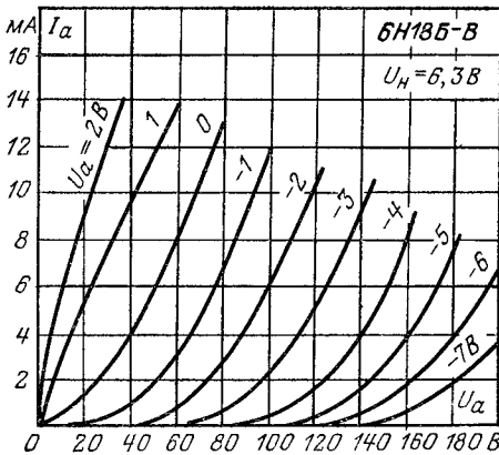
Анодные характеристики
