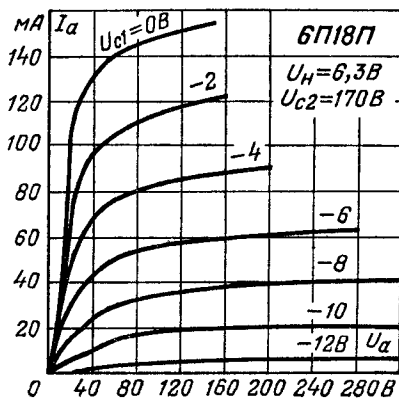
Анодные характеристики.
