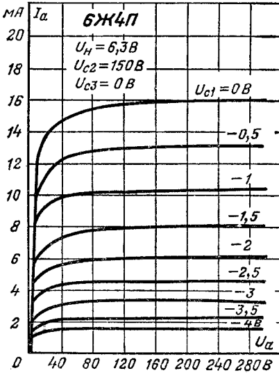
Анодные характеристики.
