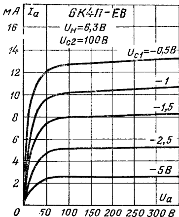
Анодные характеристики.
