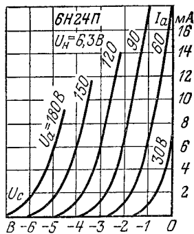
Анодно-сеточные характеристики.
