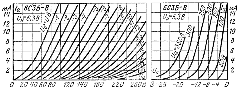
Анодные характеристики.
