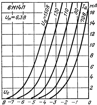
Анодно-сеточные характеристики.
