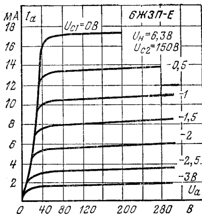
Анодные характеристики.
