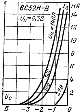
Анодно-сеточные характеристики.
