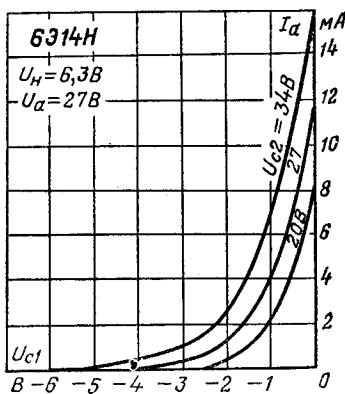
Анодно-сеточные характеристики.
