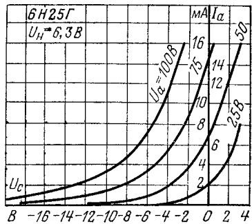
Анодно-сеточные характеристики.
