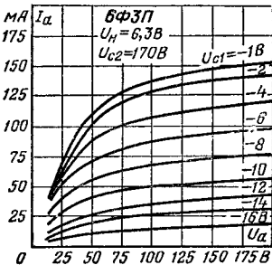
Анодные характеристики пентодной части.
