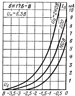
Анодно-сеточные характеристики.
