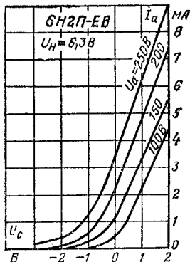
Анодно-сеточные характеристики.
