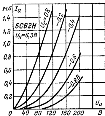
Анодные характеристики.
