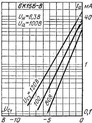
Анодно-сеточные характеристики.
