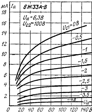
Анодные характеристики.
