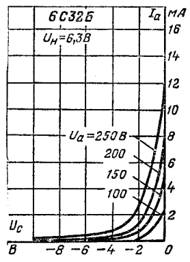
Анодно-сеточные характеристики.
