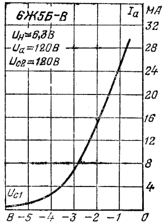
Анодно-сеточная характеристика.
